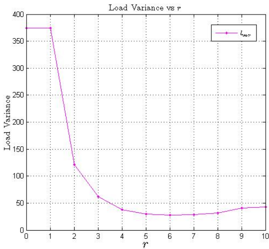
Fig. 8. Load Variance per BS vs r
